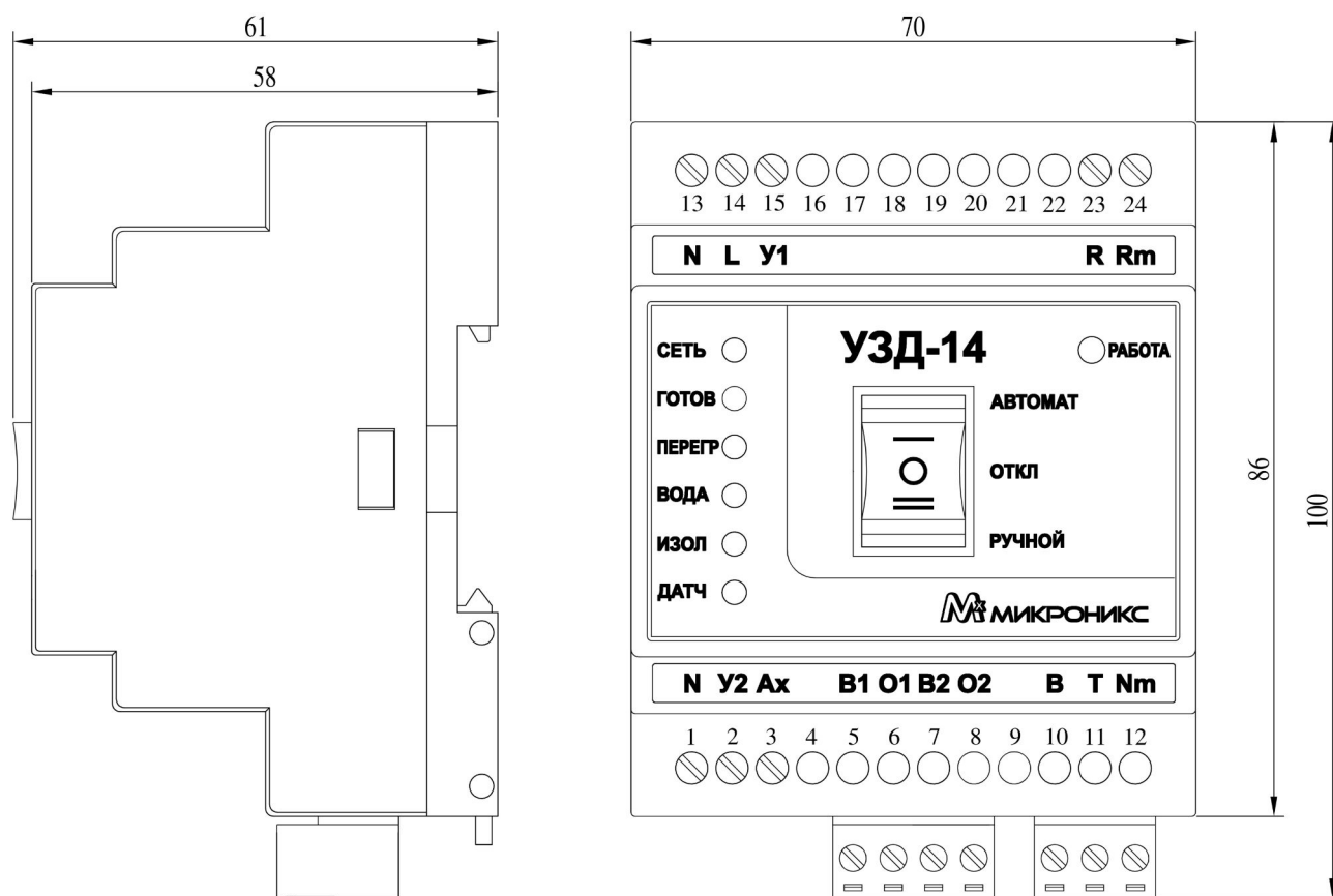
Рисунок 1 - Внешний вид устройства
