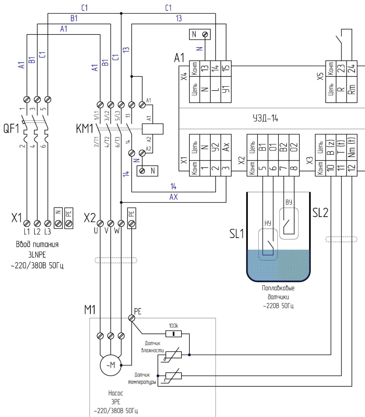
Рисунок 3 - Рекомендуемая схема включения
